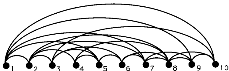
Fig. 3. Representació en fila del graf de Jayakumar.
