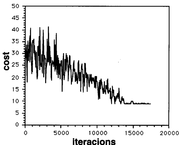
Fig. 6. Variació del cost del graf a cada iteració. Graf aleatori d'ordre 12 i 28 branques ( a = 1.13 ).
