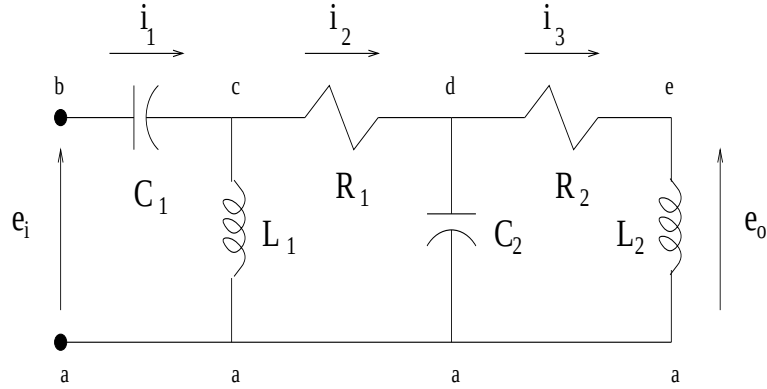
Figura 1: Circuit d'ordre 4
