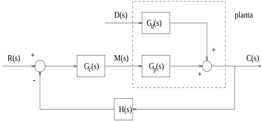
Figura 7: Un sistema de control amb pertorbacions d(t)
