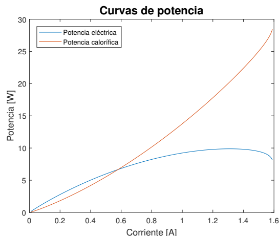
Figura 6: Curvas de potencia eléctrica y calorífica en función de la corriente de la HT-PEMFC
