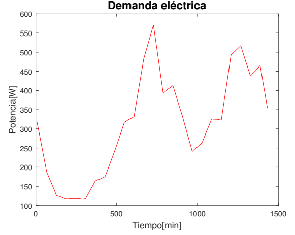
Figura 7: Demanda eléctrica para un día del mes de abril
