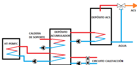
Figura 5: Esquema del sistema térmico
